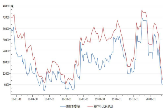
图 3：上期所铅库存
