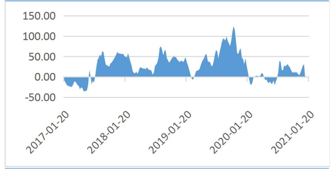
图 9：蛋鸡养殖利润
