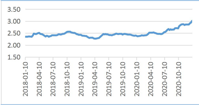
图 8：蛋鸡饲料价格
