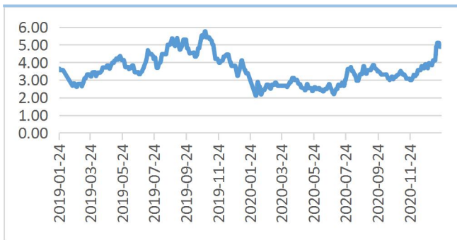
图 1：产区（河北）鸡蛋价格走势 单位：元/斤
