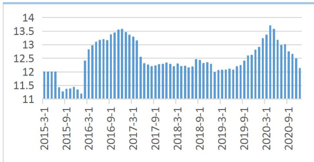
图 4：中国在产蛋鸡月度存栏量 单位：亿只
