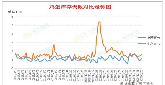
图 11：鸡蛋库存天数
