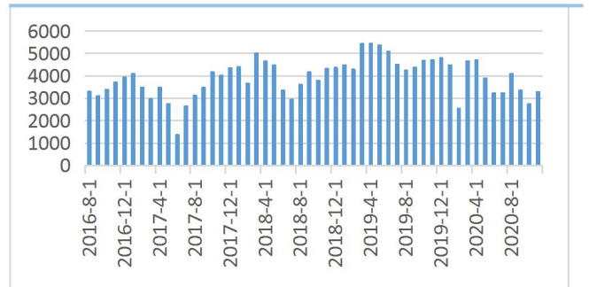
图 5：鸡苗销量 单位：万羽
