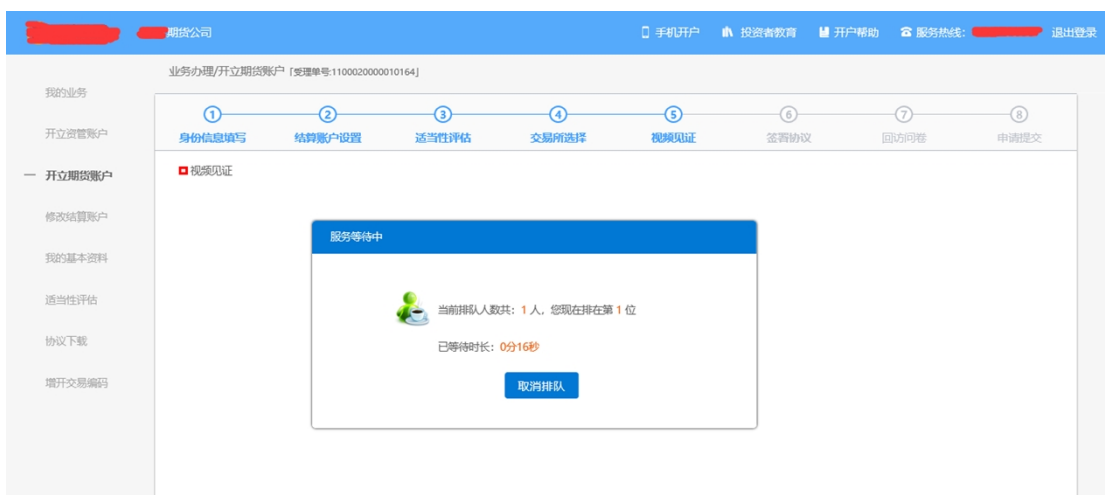
图 17 视频排队
