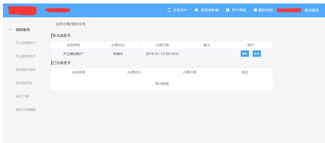
图 25 我的业务
