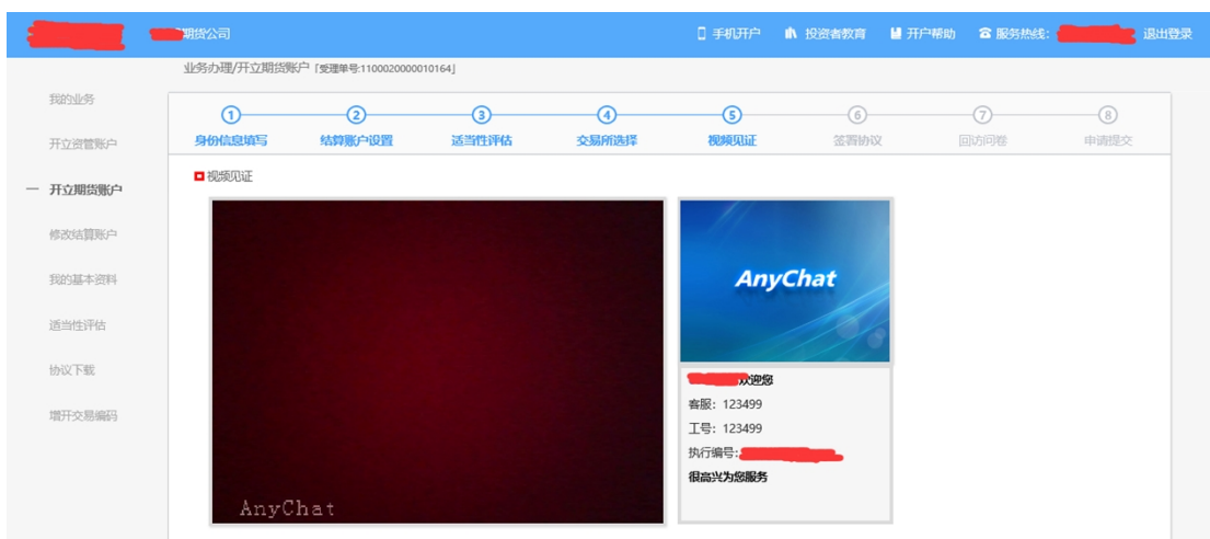
图 18 视频认证
