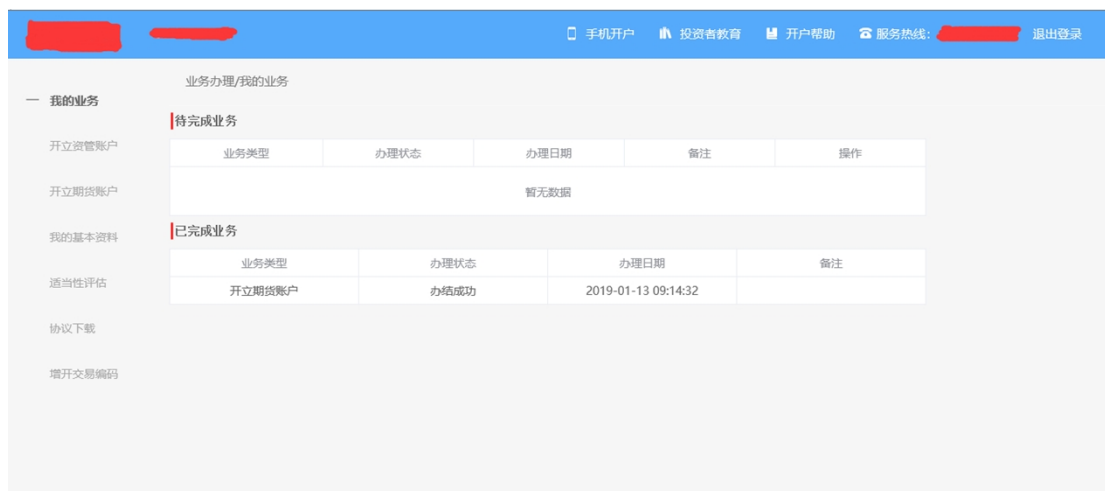
图 26 我的业务
