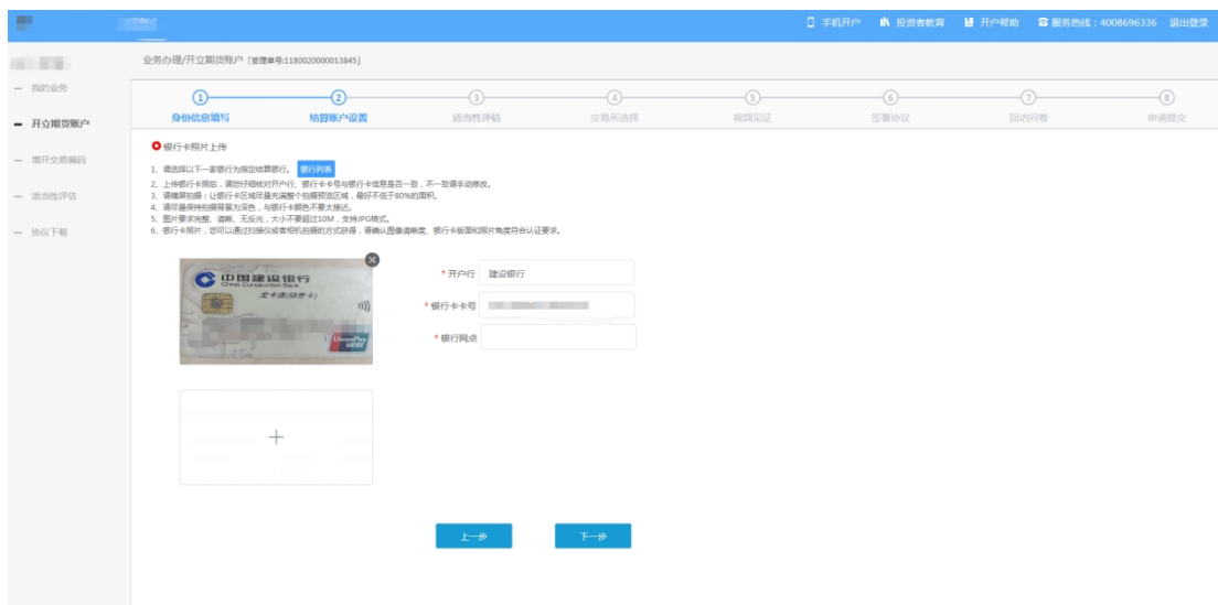
图 6 银期绑定
