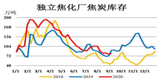
图 9：独立焦化厂焦炭库存
