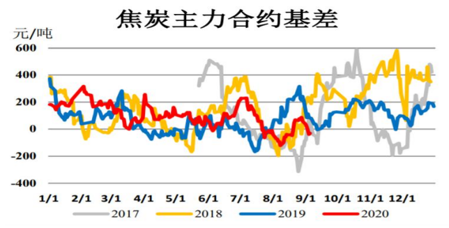
图 3：焦炭主力合约基差
