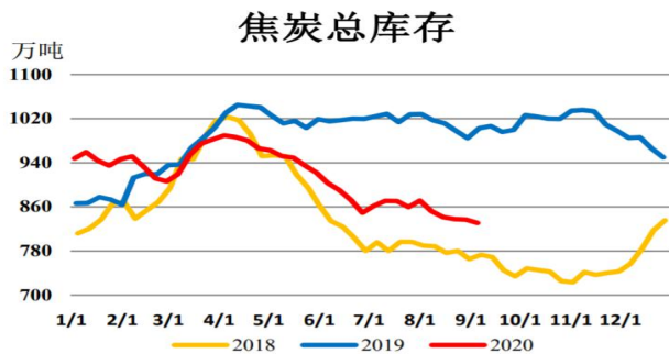
图 8：焦炭总库存
