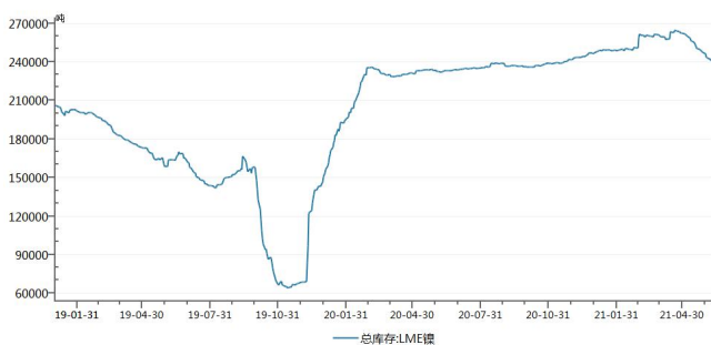
图 3：LME 镍库存
