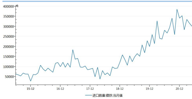
图 4：镍铁进口量
