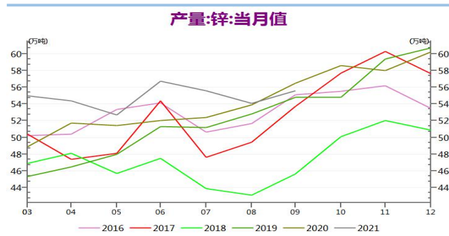
图 5：中国锌产量
