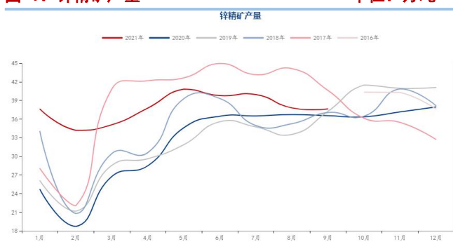
图 1：锌精矿产量
