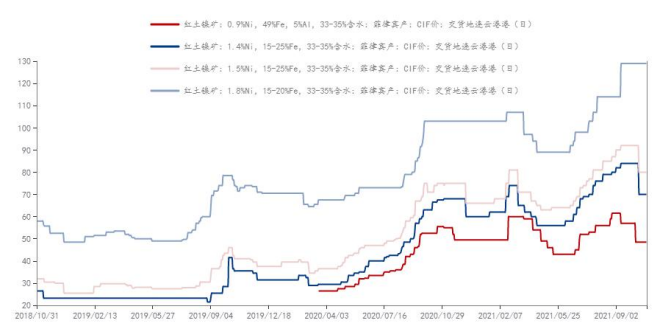
图 2：红土镍矿价格
