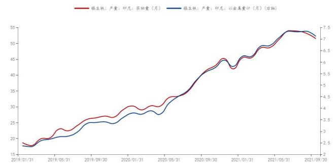
图 4：印尼镍生铁产量
